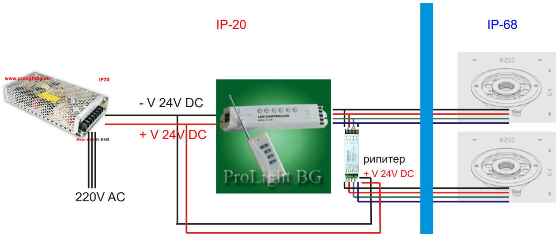
схема на свързване на захранване и контролер към светодиодни тела за вграждане във вода или настилки
